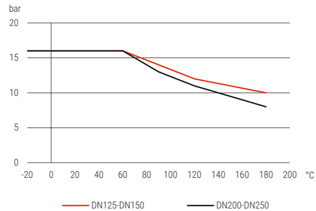
Druck-Temperatur-Diagramm pressure-temperature-diagram
